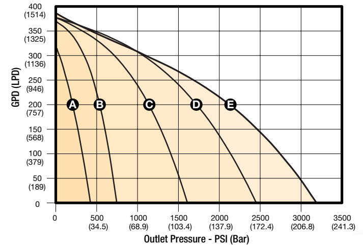
3/4" Plunger (PCI-450-75)
